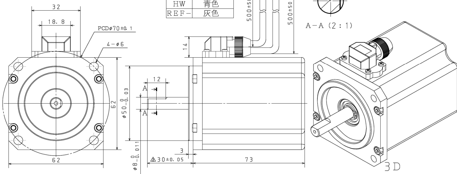
ラベル表示品番: MSH6224-170W-ST1 モータ外観: 黒色/灰色
